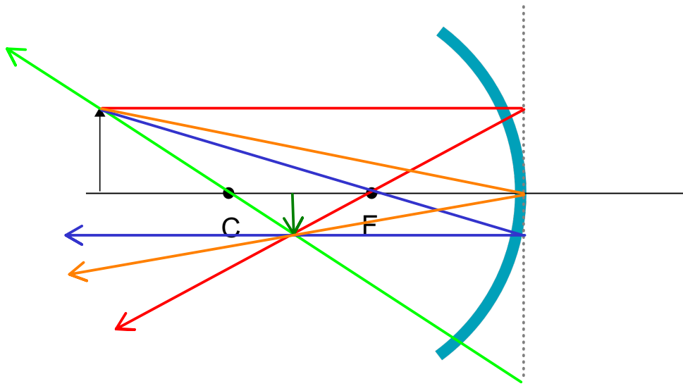
Imatge real, invertida i menor
